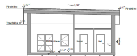
Schnitt AA
