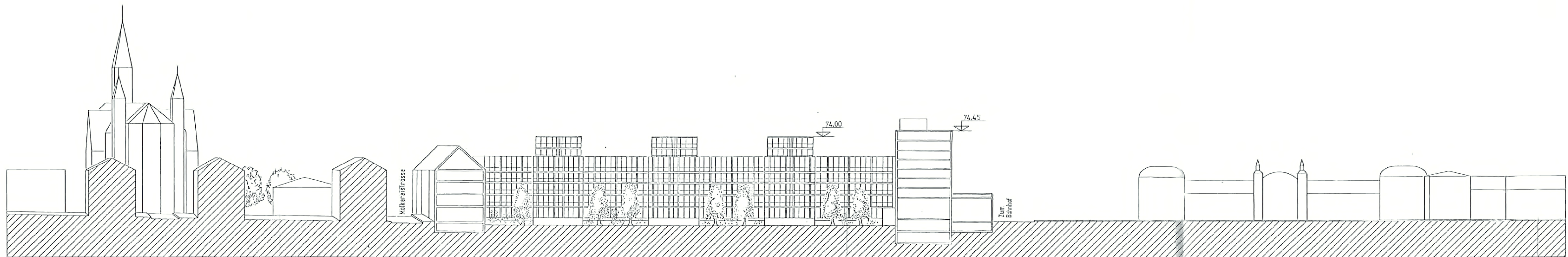
SCHNITT A-A
