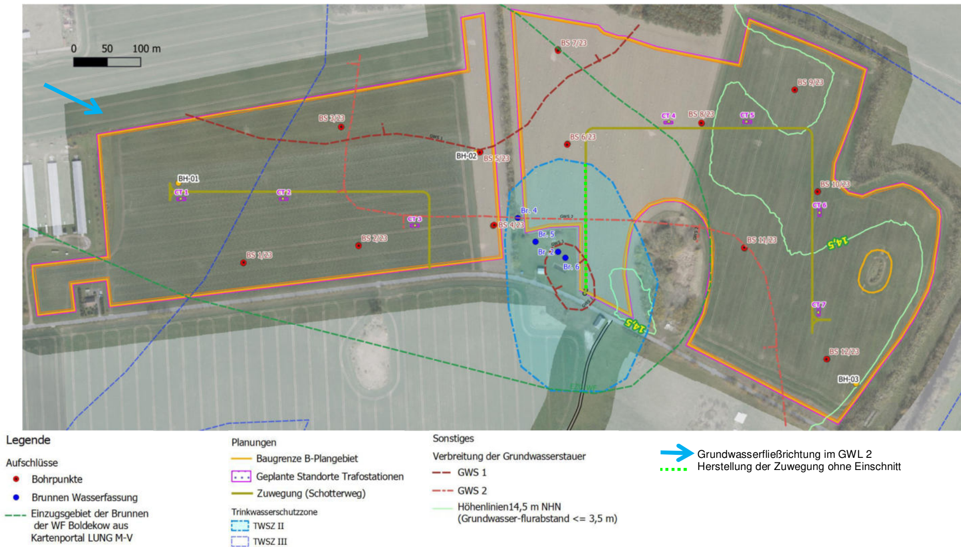
Abbildung 4: Bauliche Maßnahmeempfehlungen zum Grundwasserschutz im B-Plangebiet
