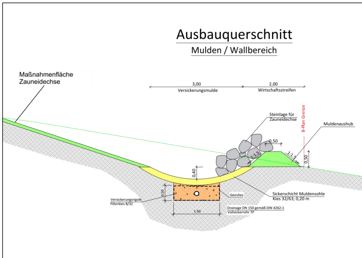
Abb. 4: Technische Vorplanung im Ausbauquerschnitt für die Versickerungsmulde und das Zauneidechsen-Ersatzquartier (Ing.-Büro Möller, Grevesmühlen, Feb. 2023)
