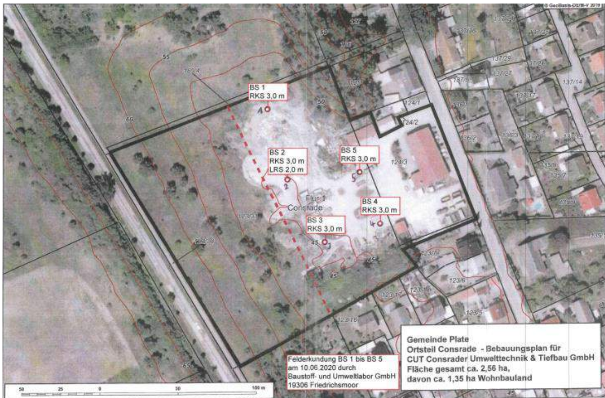
Abb. 6: Lage der Erkundungsstellen (Karte aus dem Bericht zur Baugrundbegutachtung 14.08.2021)
