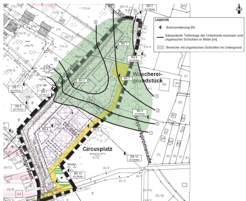
Abbildung 4: Baugrund, Bodengutachten [1]
