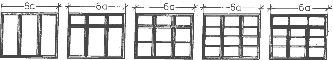
Liegende, große Fenster
