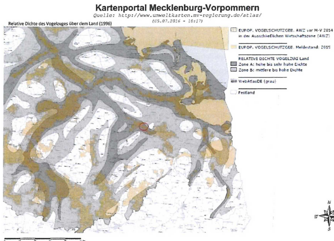
Abbildung 3: Relative Dichte des Vogelzuges über dem Land ( www.umweltkarten.mv-regierung.de )
