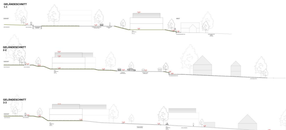
Abbildung 5: Beispielhafte Geländeschnitte zur Entwicklung der Flächen der ehemaligen Gärtnerei (A&P Wismar, 10.10.2024).
