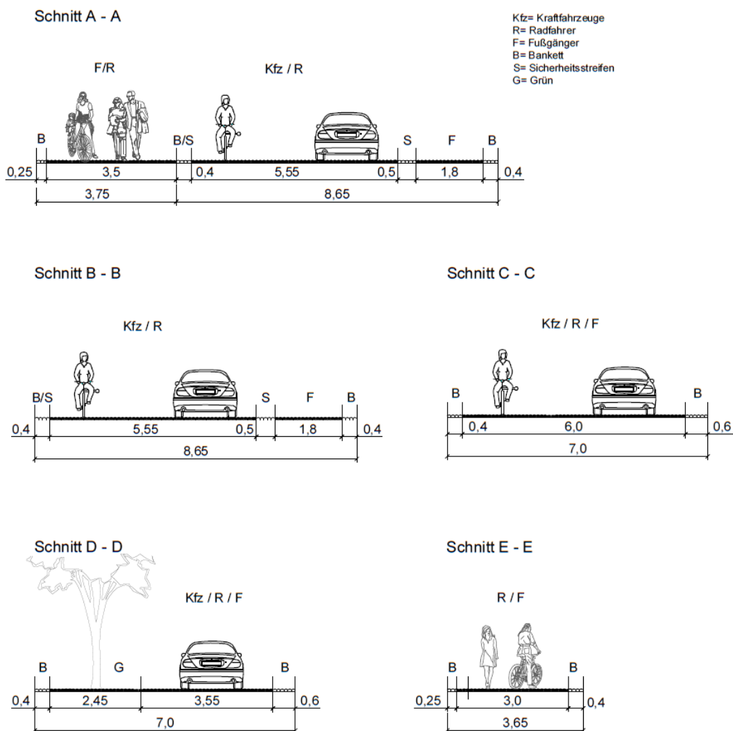
Abbildung 7: Empfohlene Straßenquerschnitte
