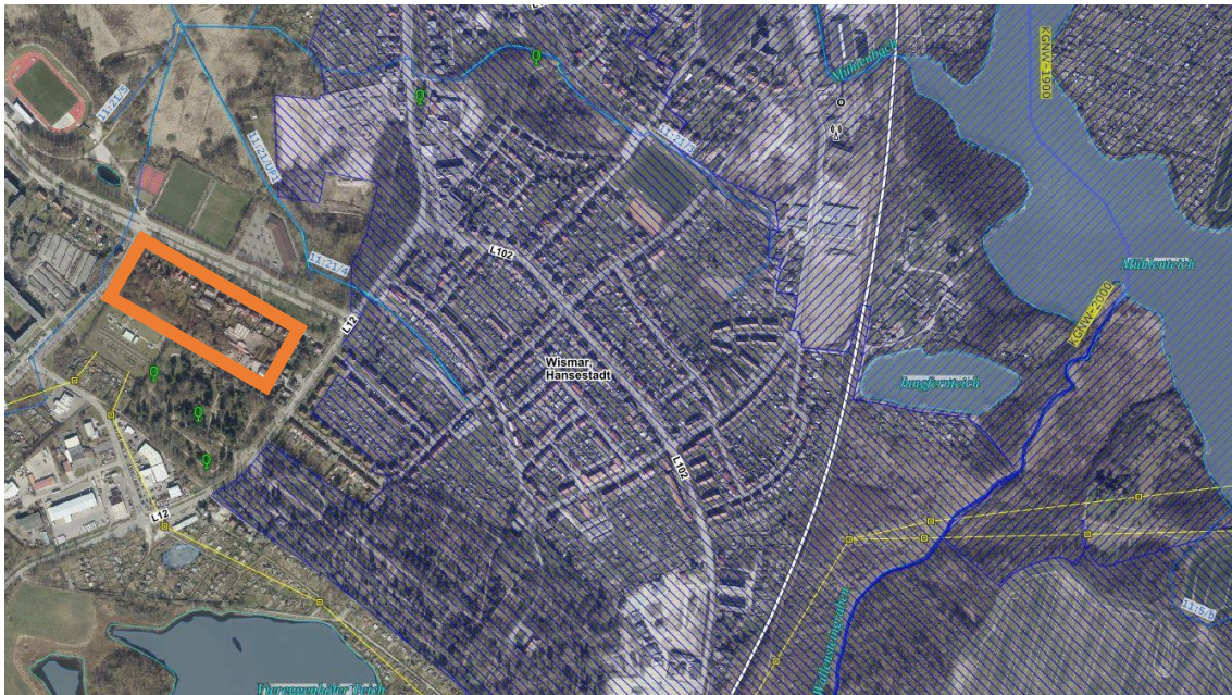
Abbildung 13: Darstellung der Wasserschutzgebiete III Wismar-Friedrichshof (blau gestreifte Flächen) in der Nähe des Planbereiches (orangene Umrahmung) (Geodatenportal M-V 2022).
