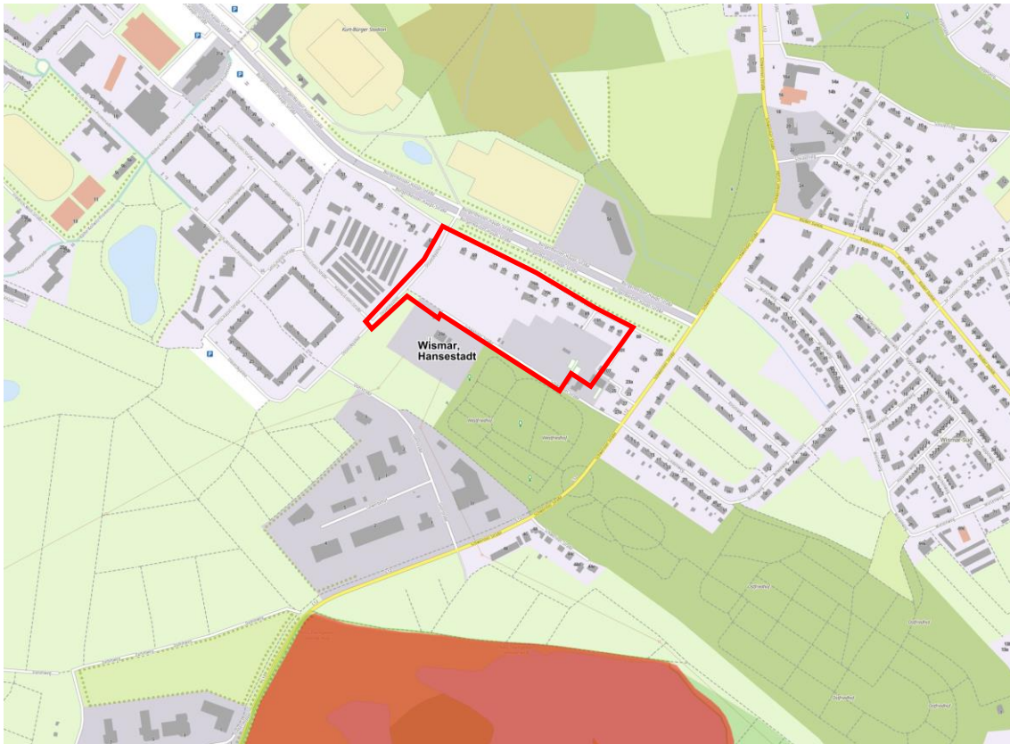
Abbildung 11: Nationale Schutzgebiete (LSG und NSG als rote Fläche dargestellt) südlich vom Plangebiet (rote Umgrenzung). Quelle: GAIA M-V 202
