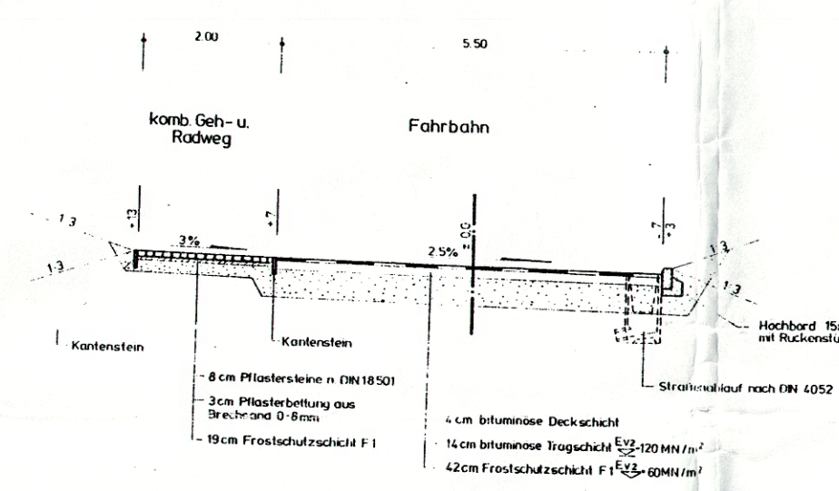
Planstraße Schnitt B M 1:100
