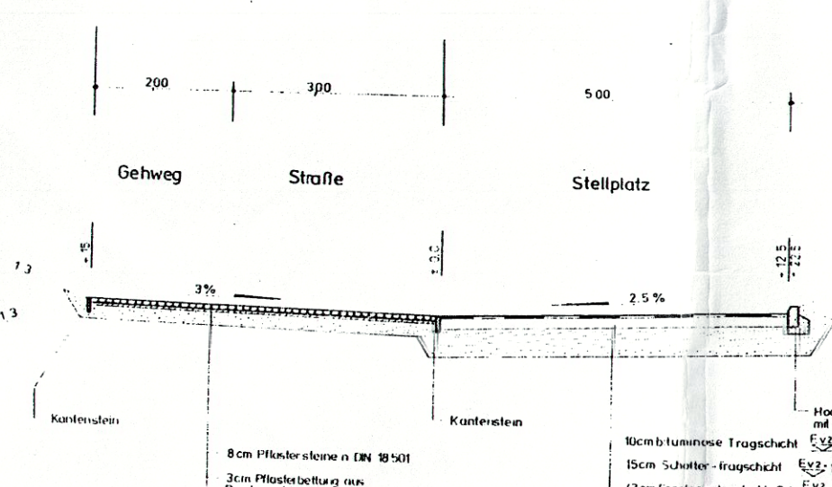
Planstraße Schnitt C M 1:100
