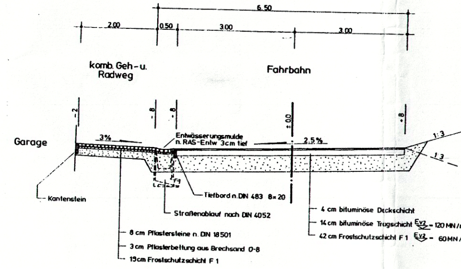
Planstraße Schnitt A M 1:100
