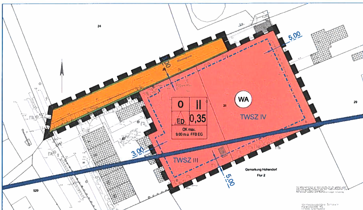
Abb. 2 Planzeichnung
