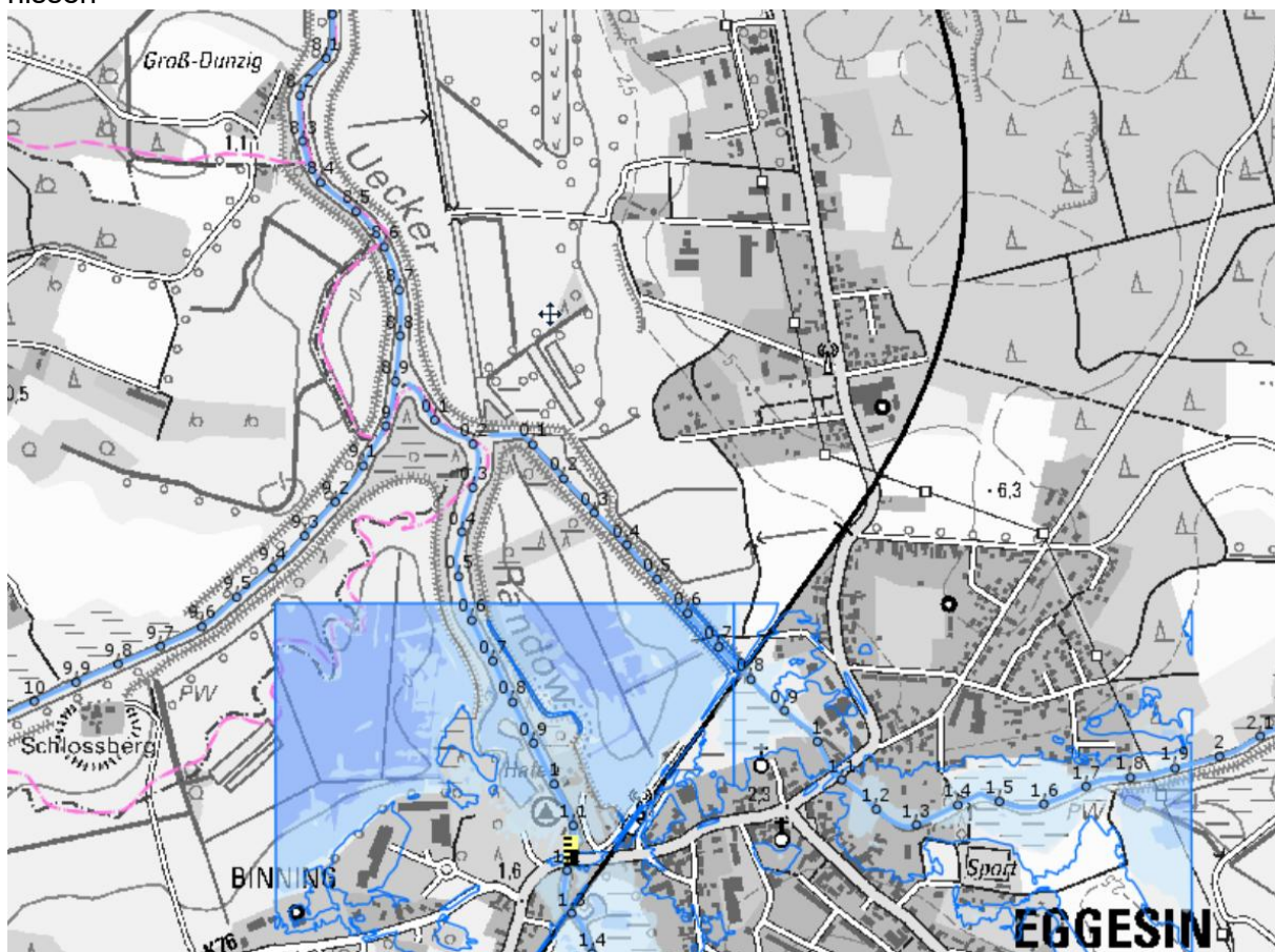
Abbildung 3: Plangeltungsbereich mit überflutungsgefährdeten Bereichen bei Extremereignissen
