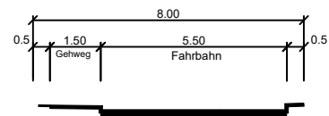
STRÄßENQUERSCHNITT SCHNITT A - A
