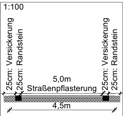
Planstraße D (Lindenweg) Straßenschemaquerschnitt
