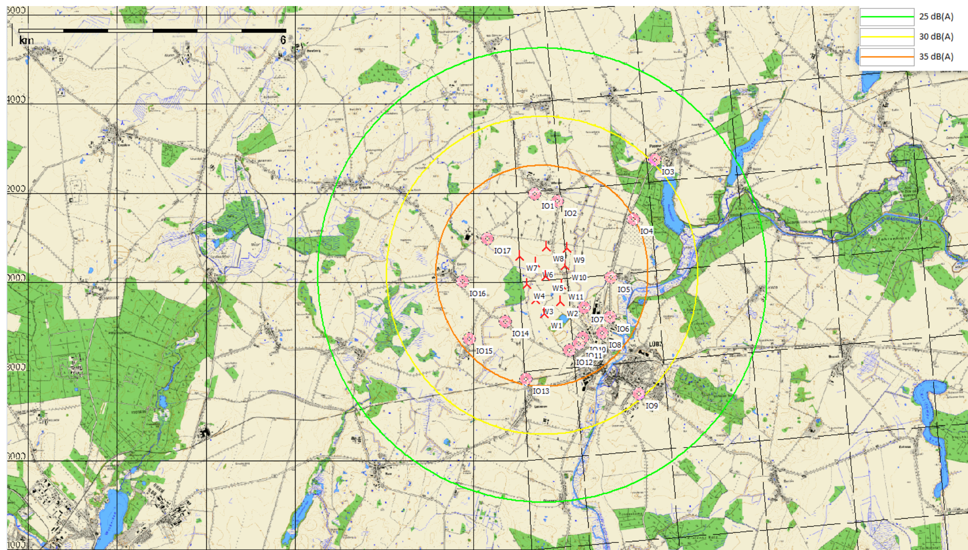
Abbildung 9.3: Einwirkungsbereich Schall – Isolinien (nachts), Standort Werder/Lübz
