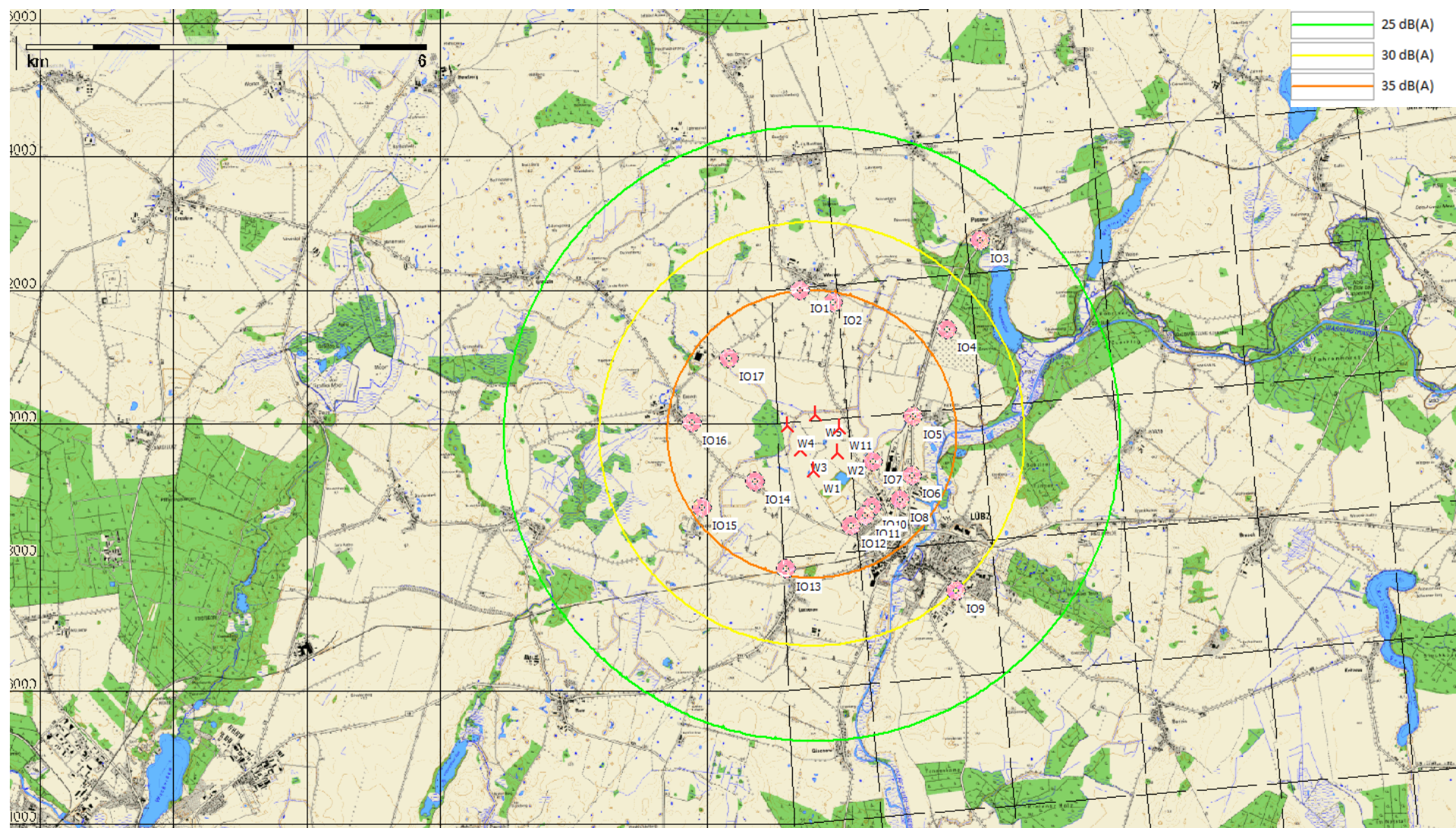
Abbildung 9.2: Einwirkungsbereich Schall – Isolinien (nachts), Standort Lübz
