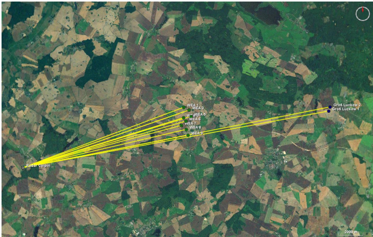
Abbildung 2: Luftaufnahme des Windparks Badresch mit den geplanten Windenergieanlagen (grün), sowie der berücksichtigten Vorbelastung (blau). Die Einstrahlungsrichtungen bzgl. der Radaranlage Cölpin sind gelb dargestellt.
