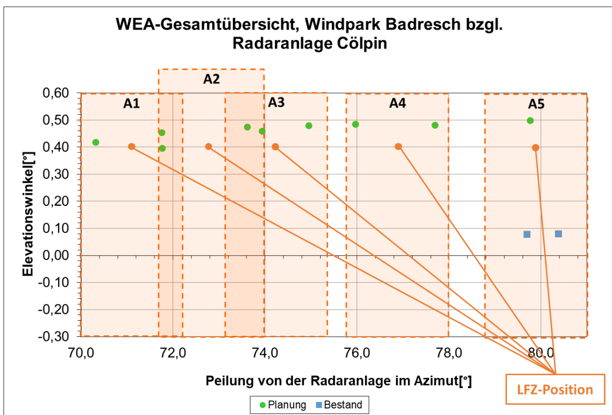
Abbildung 12: Perspektive zur Gondelanordnung gemäß Azimut und Elevation für die Position des Radars Cölpin. Die Bereiche der analysierten Teilanordnungen sind durch farbige Flächen gekennzeichnet. Die Richtung und Elevation des angenommenen Lfz ist dargestellt.
