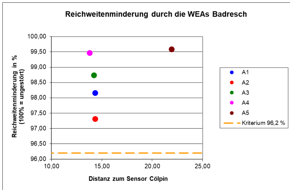
Abbildung 11: Übersicht über die zu erwartende Reichweitenreduktion bei den angegebenen WEA-Konstellationen
