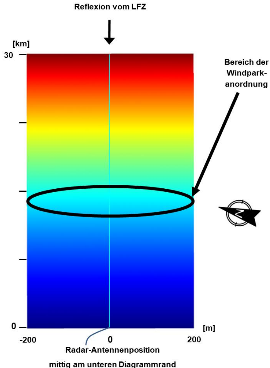
Abbildung 4: Feldgebiet von 30 km x 400 m in der Übersicht (schematische Übersicht für das Radar Cölpin)
