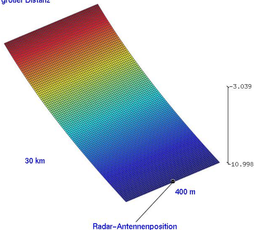
Abbildung 5: Das dargestellte Raumgebiet mit einer Elevation von 0,4° ohne WEA-Einfluss in der Konturdarstellung für die Betriebsfrequenz des Radars Cölpin
