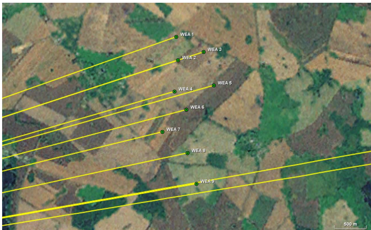
Abbildung 13: Übersicht über den Windpark Badresch mit den geplanten Windenergieanlagen (grün) sowie der berücksichtigten Vorbelastung (blau). Die Einstrahlungsrichtungen bzgl. der Radaranlage Cölpin sind gelb dargestellt.
