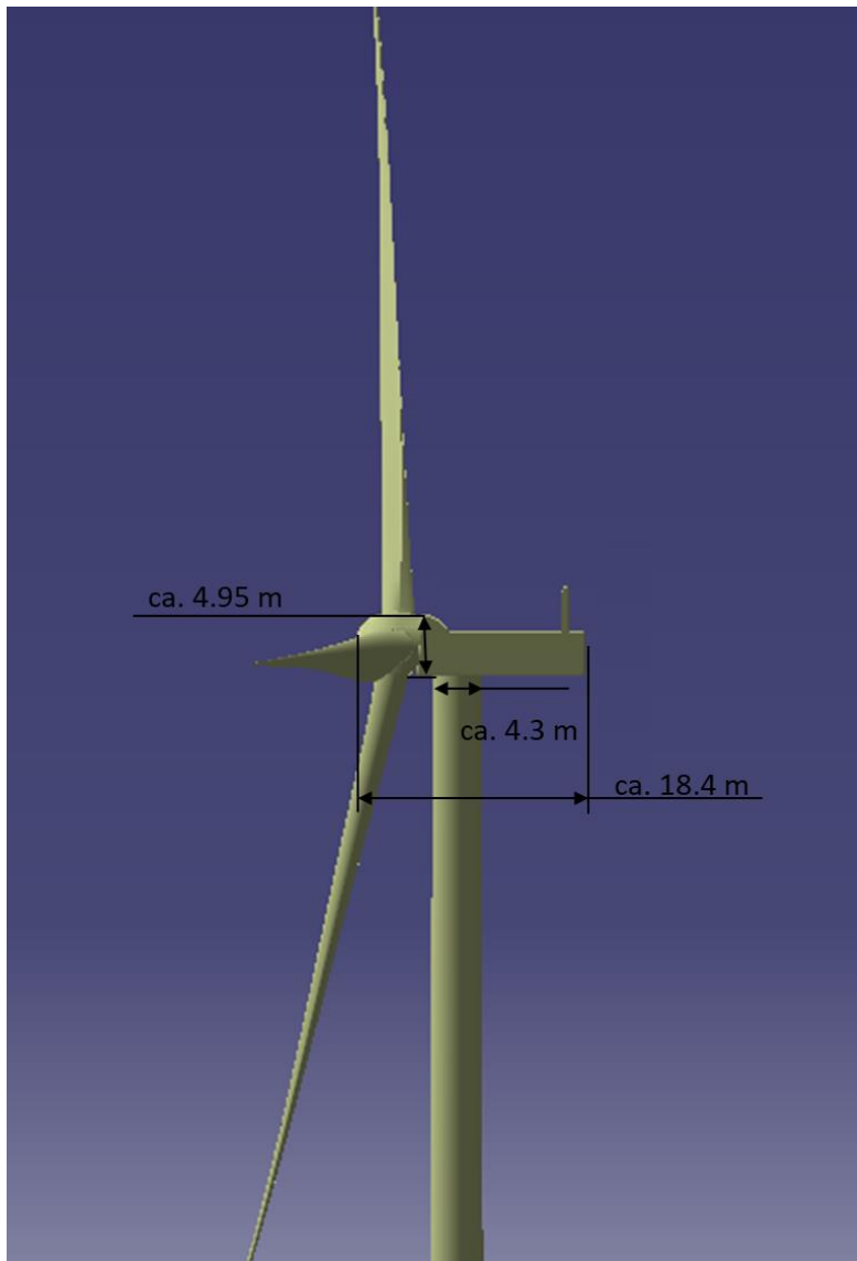
Abbildung 1: Schematische Objektgeometrie für die geplante WEA-Bauform Vestas V162 mit ca. 162 m Rotor
