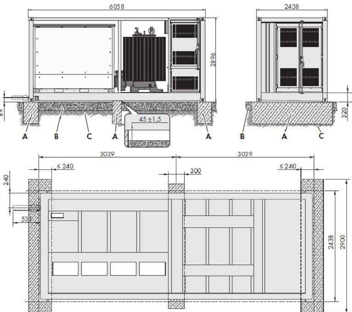
Abbildung 40: Aufstellvariante mit Stellerfundamenten (Maßangaben in mm)
