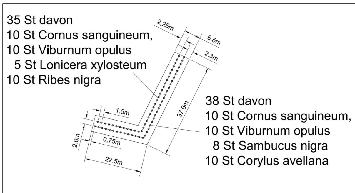
Abb. 11: Pflanzschema Hecke
