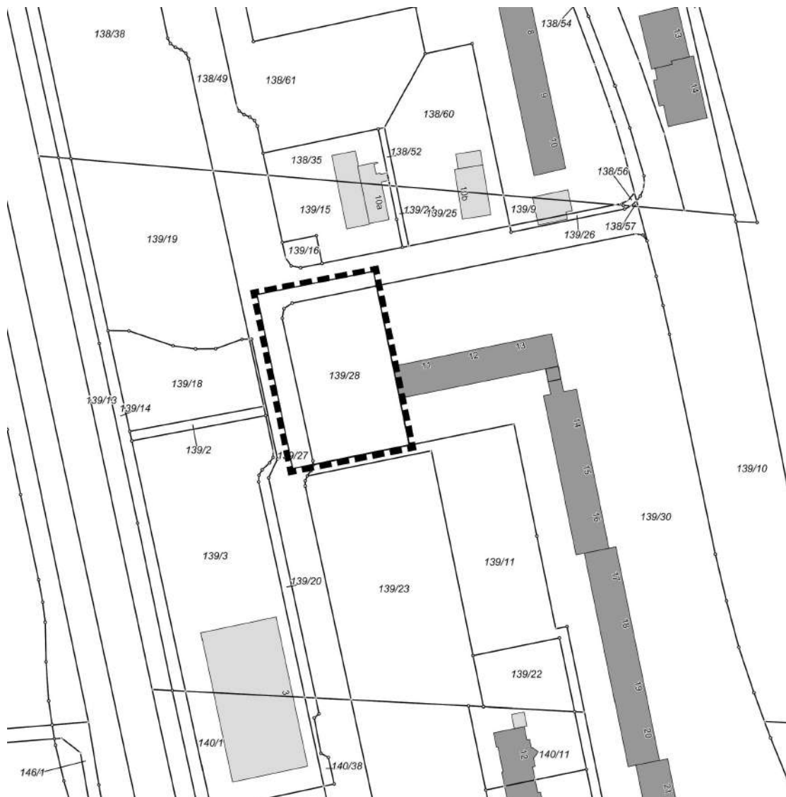
Lageplan zur 7. Änderung des Bebauungsplanes Nr. 2A der Gemeinde Saal
