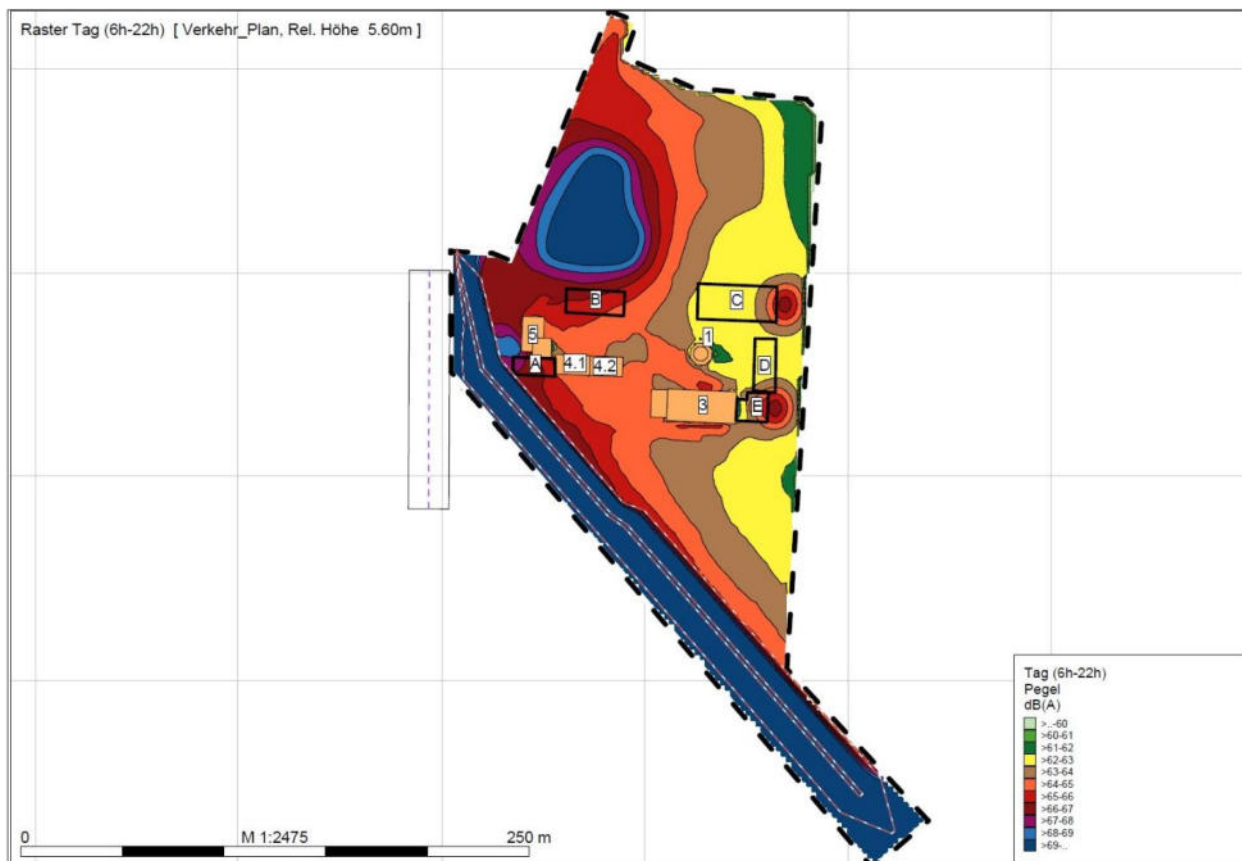
Abbildung 11: Ergebnisse der Rasterberechnung maßgeblicher Außenlärmpegel Tag
