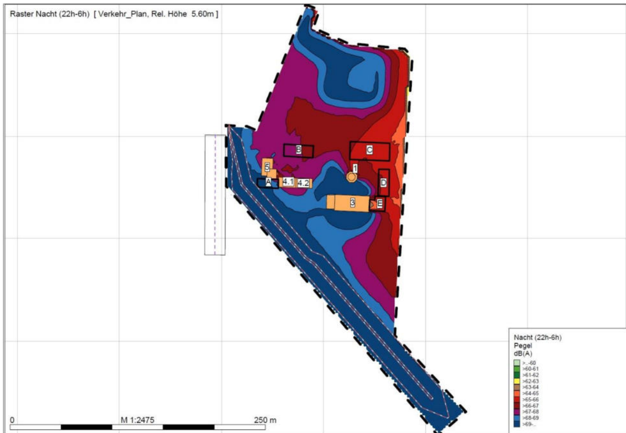
Abbildung 12: Ergebnisse der Rasterberechnung maßgeblicher Außenlärmpegel Nacht
