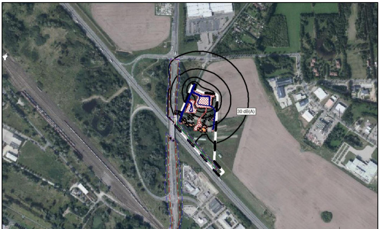
Abbildung 9: Ergebnisse der Rasterberechnung für Zusatzbelastung durch gewerbliche Anlage im Geltungsbereich des B-Planes (Nacht 22:00 Uhr – 6:00 Uhr) BA2 Bistro
