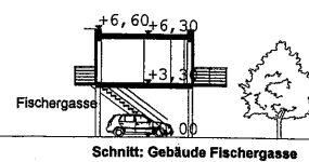
Schnitt: Gebäude Fischergasse
