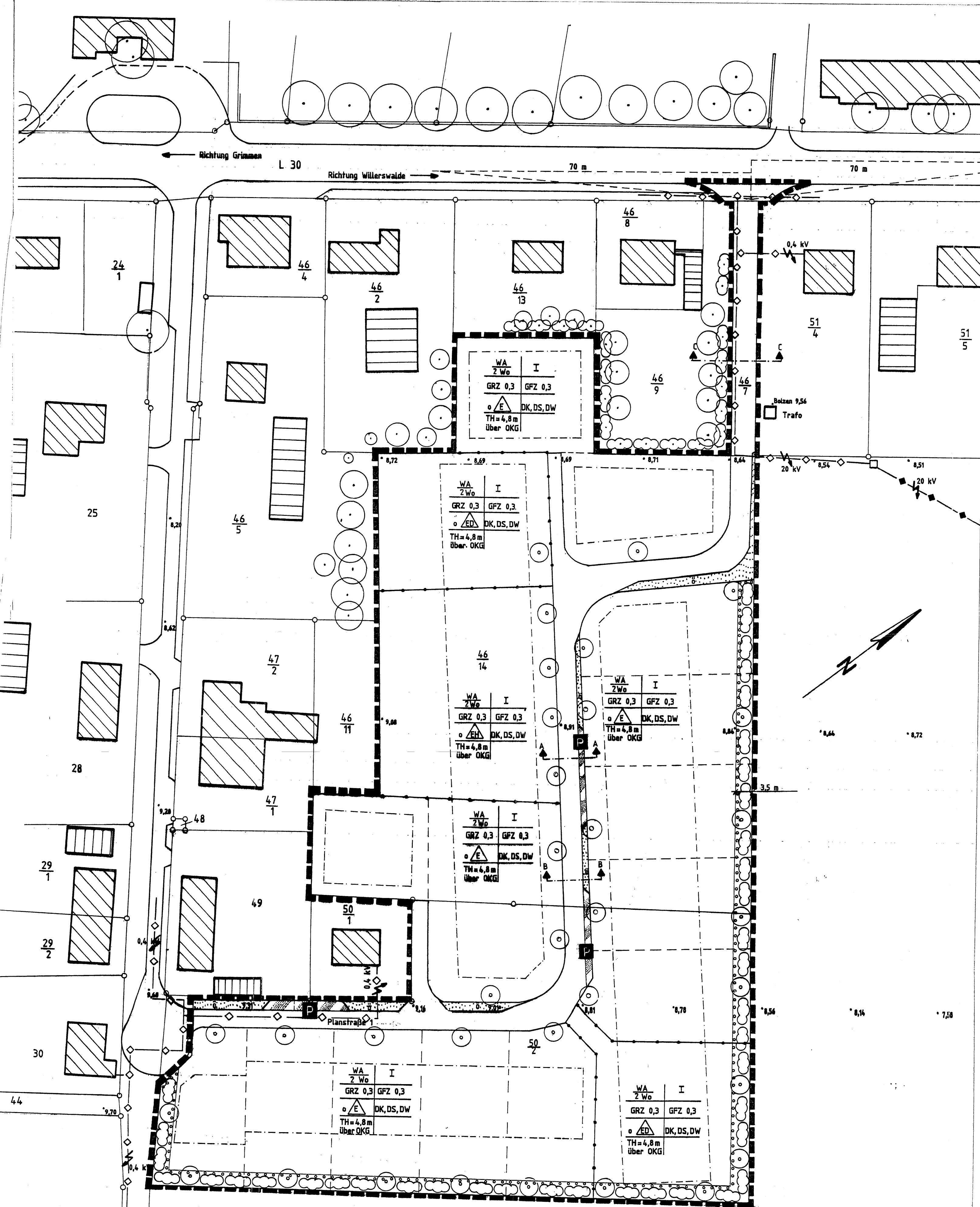
TEIL A - PLANZEICHNUNG M 1 : 500
