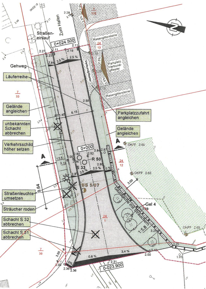
Draufsicht, M. 1:200
