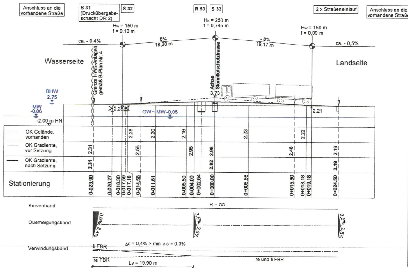
Höhenplan, M. 1:200
