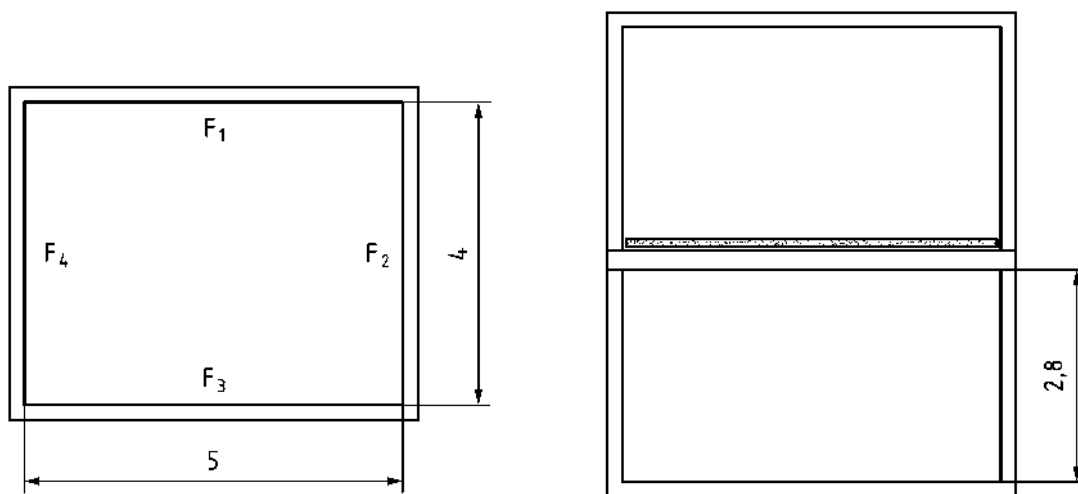
Bild D.3 — Grundriss (links) und Schnitt (rechts) zweier übereinanderliegender Räume im Holzbau (Prinzipiskizze)
