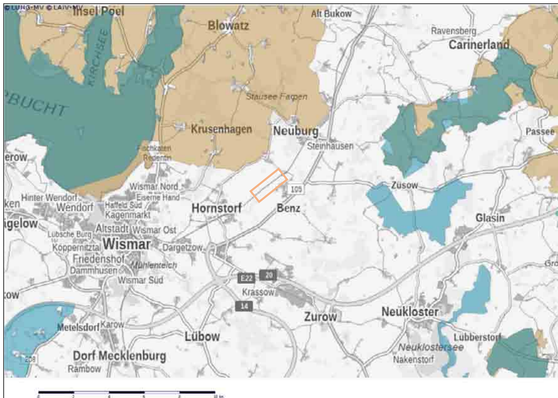
Abbildung 6: Nationale und internationale Schutzgebiete im Umfeld des Plangebietes (orange). Karte erstellt mit QGIS 3.16, Kartengrundlage: Topografische Karte LAIV-MV 2022.
