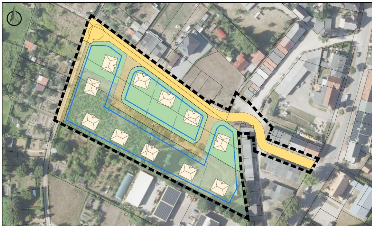
Abbildung 4: Städtebaulicher Entwurf
